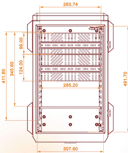
Bottom
