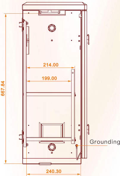
Inner Left
